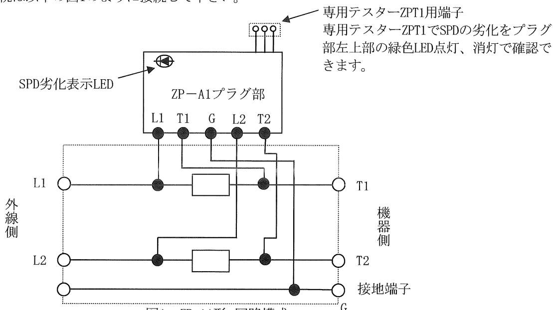
図1. ZP-A1形 回路構成
