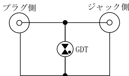
図1 回路構成
