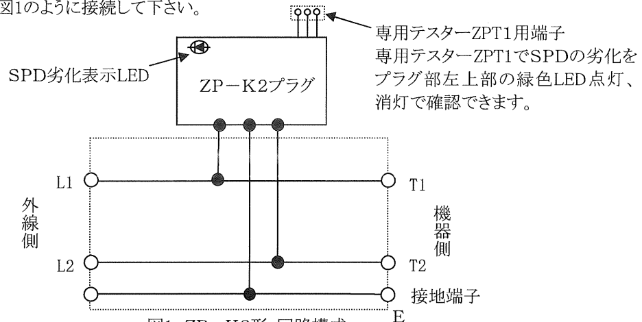
図1. ZP-K2形 回路構成
