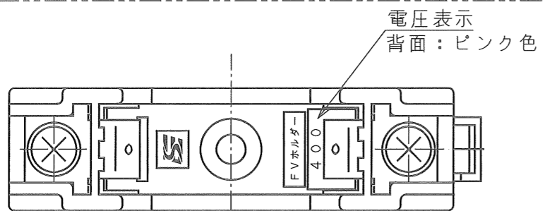
保安器本体
