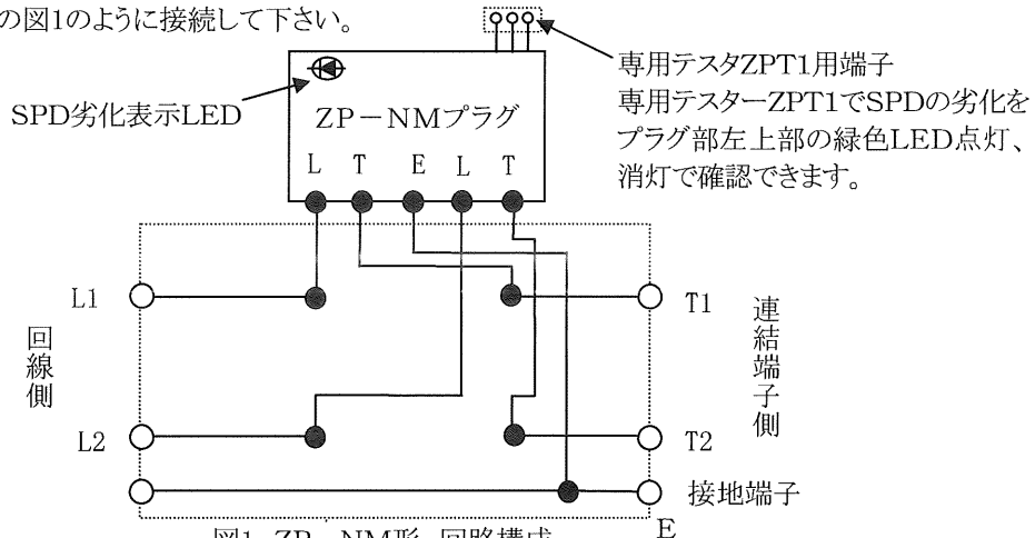
図1. ZP-NM形 回路構成
