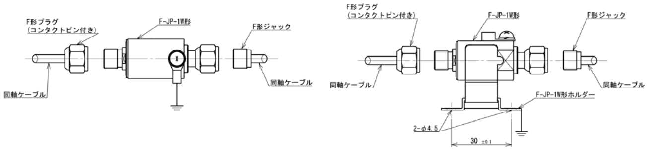
図2 同軸ケーブルの中間に接続する取付方法
