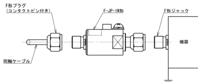
図1 本製品を機器へ直接接続する取付方法
