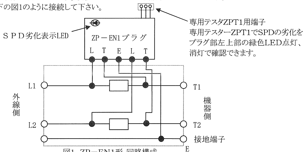
図1. ZP-EN1形 回路構成
