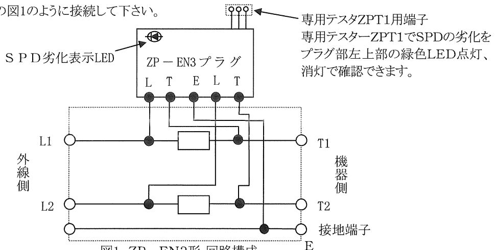
図1. ZP-EN3形 回路構成
