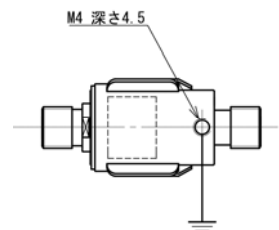
図3 ねじ穴を利用する場合
