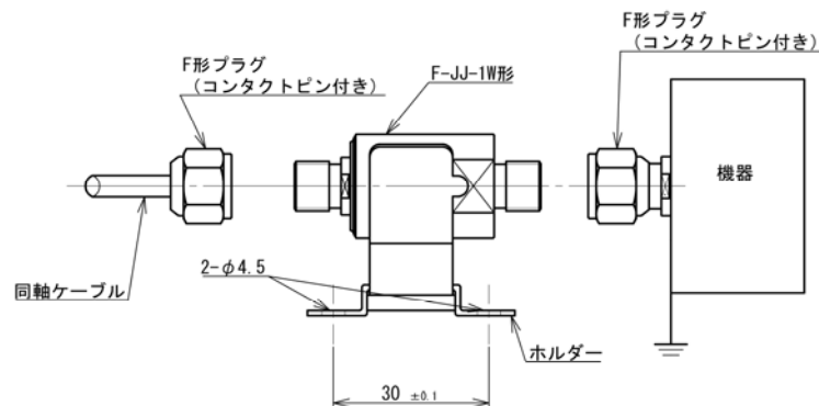
図1 本製品を機器へ直接接続する取付方法
