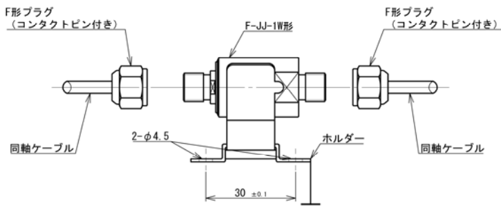
図2 同軸ケーブルの中間に接続する取付方法
