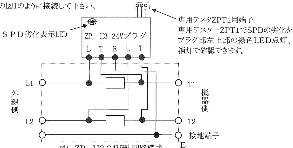
図1. ZP-H3 24V形 回路構成
