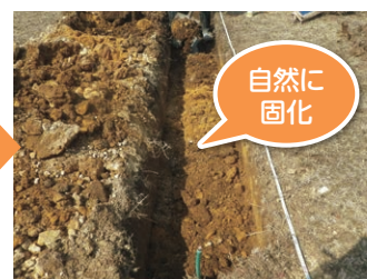
④埋戻し
