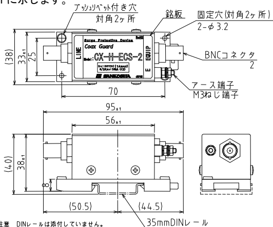
図1 外観図
